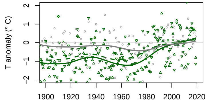
MAM
