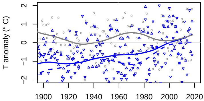
DJF
